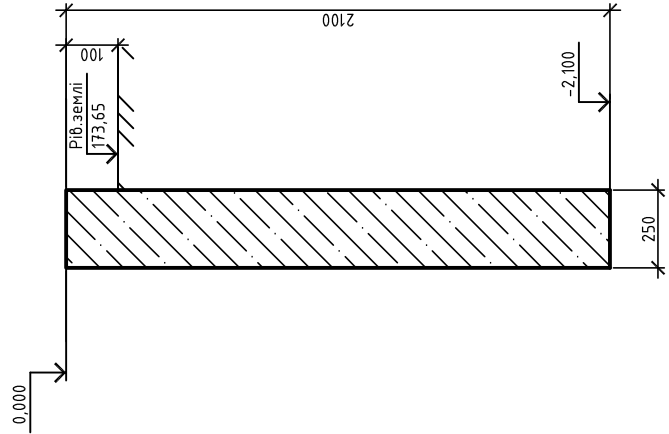
1-1 (опалубка)
