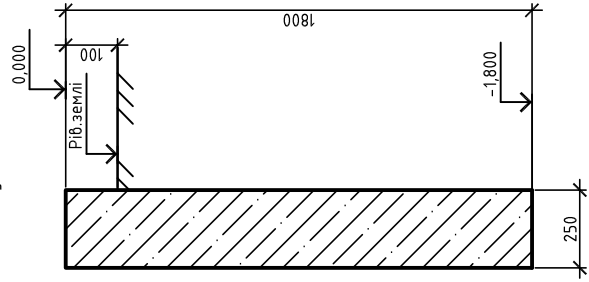
2-2 (опалубка)
