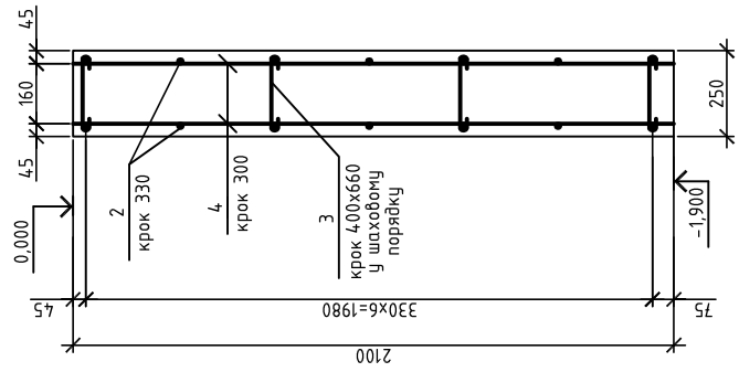
1-1 (армування)
