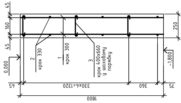
2-2 (армування)
