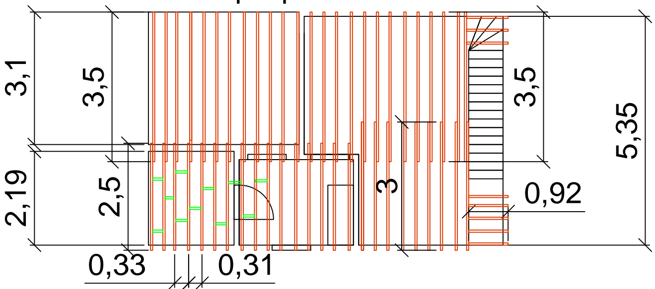
План балок перекрытия
