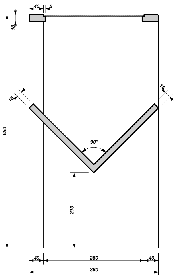
Разрез
